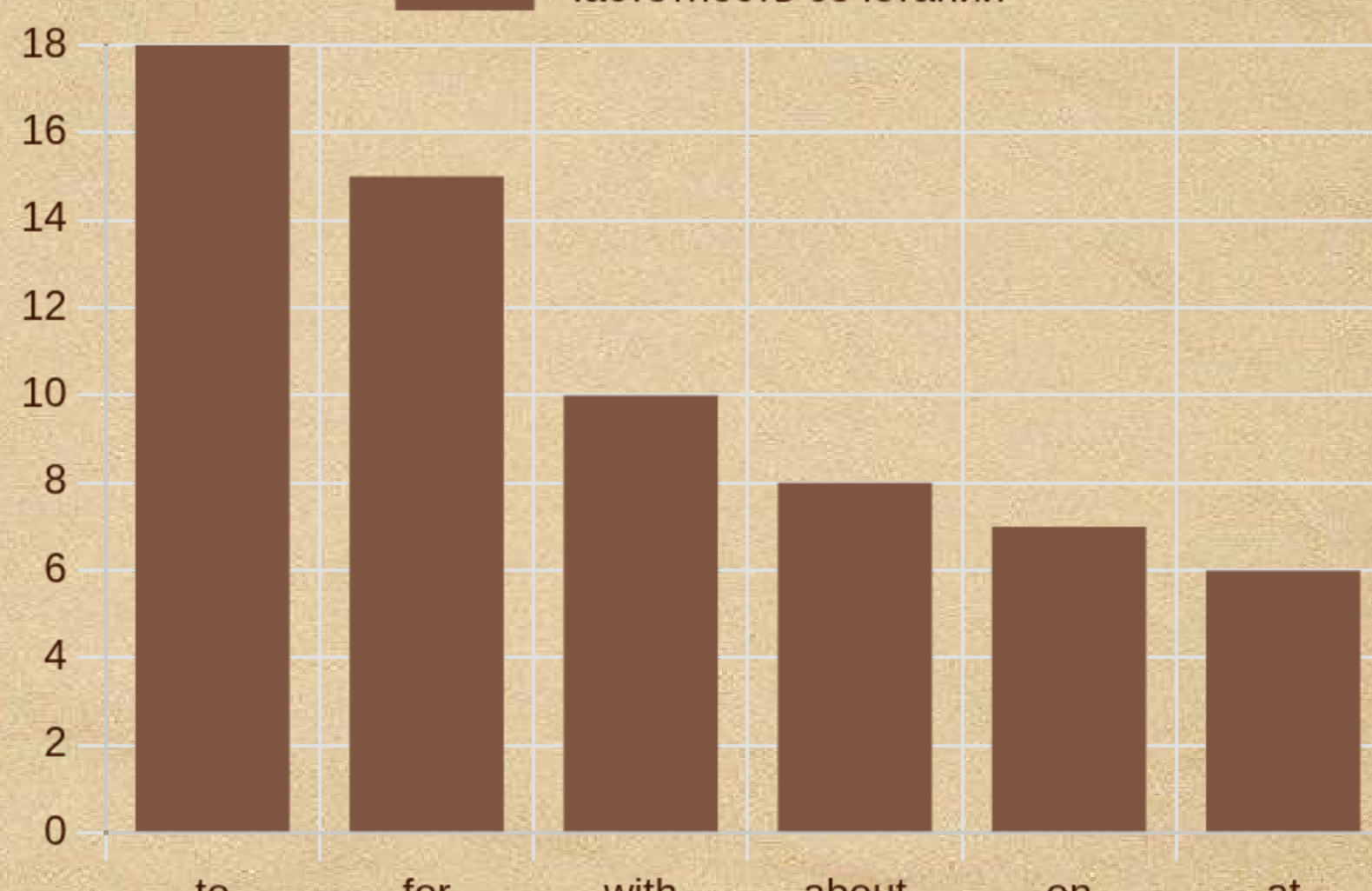
Частотность сочетаний
